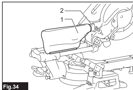
Fig.34 ► 1. Bolsa recolectora de polvo 2. Boquilla para polvo
