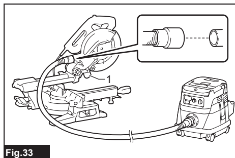
Fig.33 ► 1. Protector de recolección de polvo
